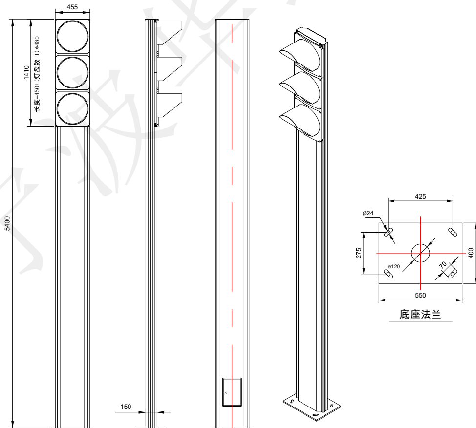
400一体化灯杆尺寸图
