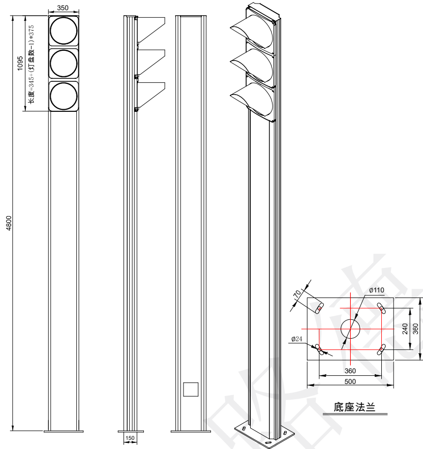
300一体化灯杆尺寸图
